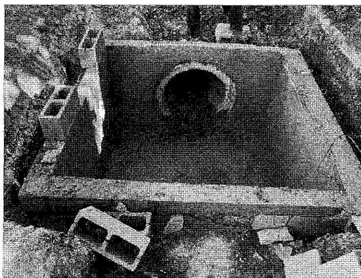
Assentamento tubulação de 500mm
