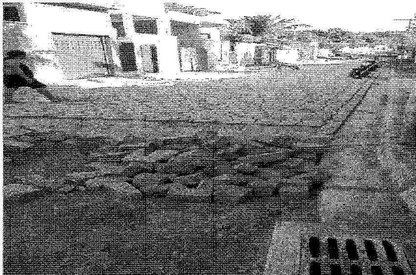
Execução de sub-base
