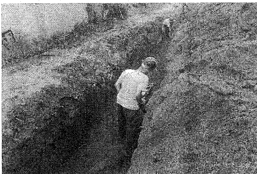
Assentamento e Embasamento de Tubulação.
