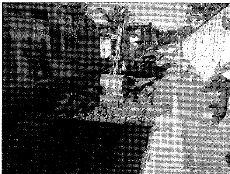
Retirada de material para execução de sub-base
